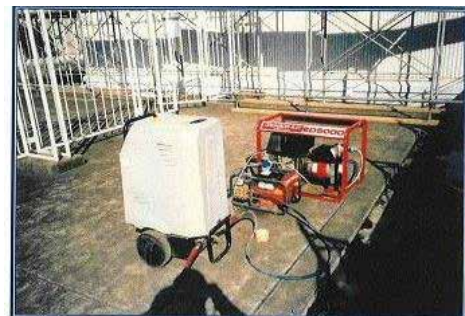
コンプレッサ、高効率ボイラー、 発電機によるコンパクトシステム
